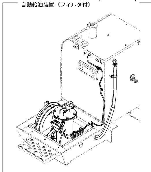
AUTO FUEL FILLING DEVICE (WITH FILTER) 自動給油装置（フィルタ付）
