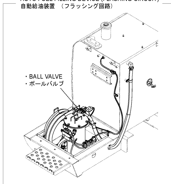
AUTO FUEL FILLING DEVICE (FLASHING CIRCUIT) 自動給油装置（フラッシング回路）
