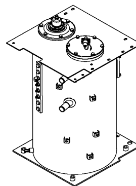
OIL TANK (WITH INDICATOR) オイルタンク (インジケータ付)
